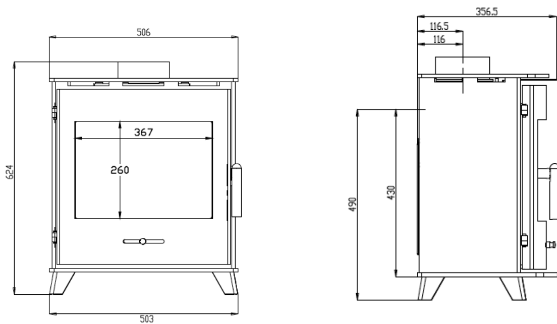
Technický výkres hede 4:
