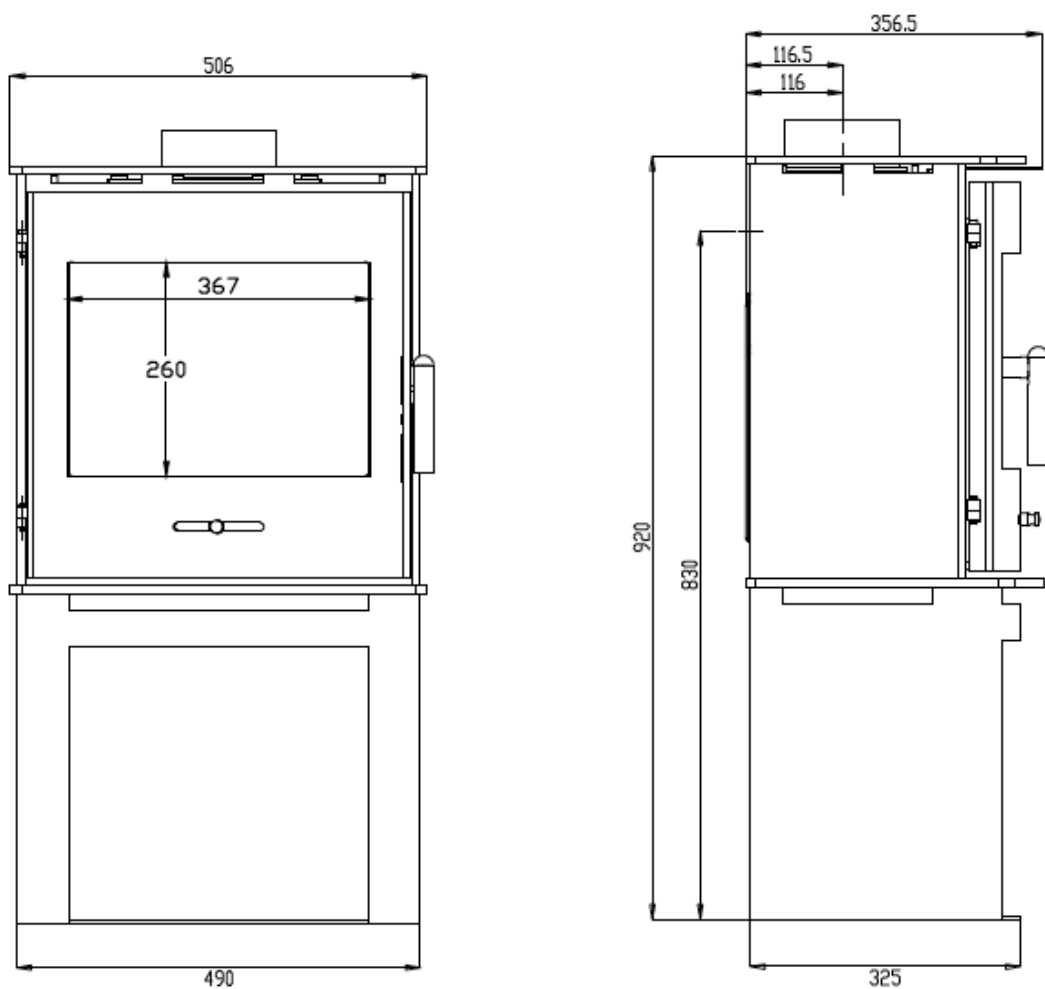
Technický výkres hede 4D:
